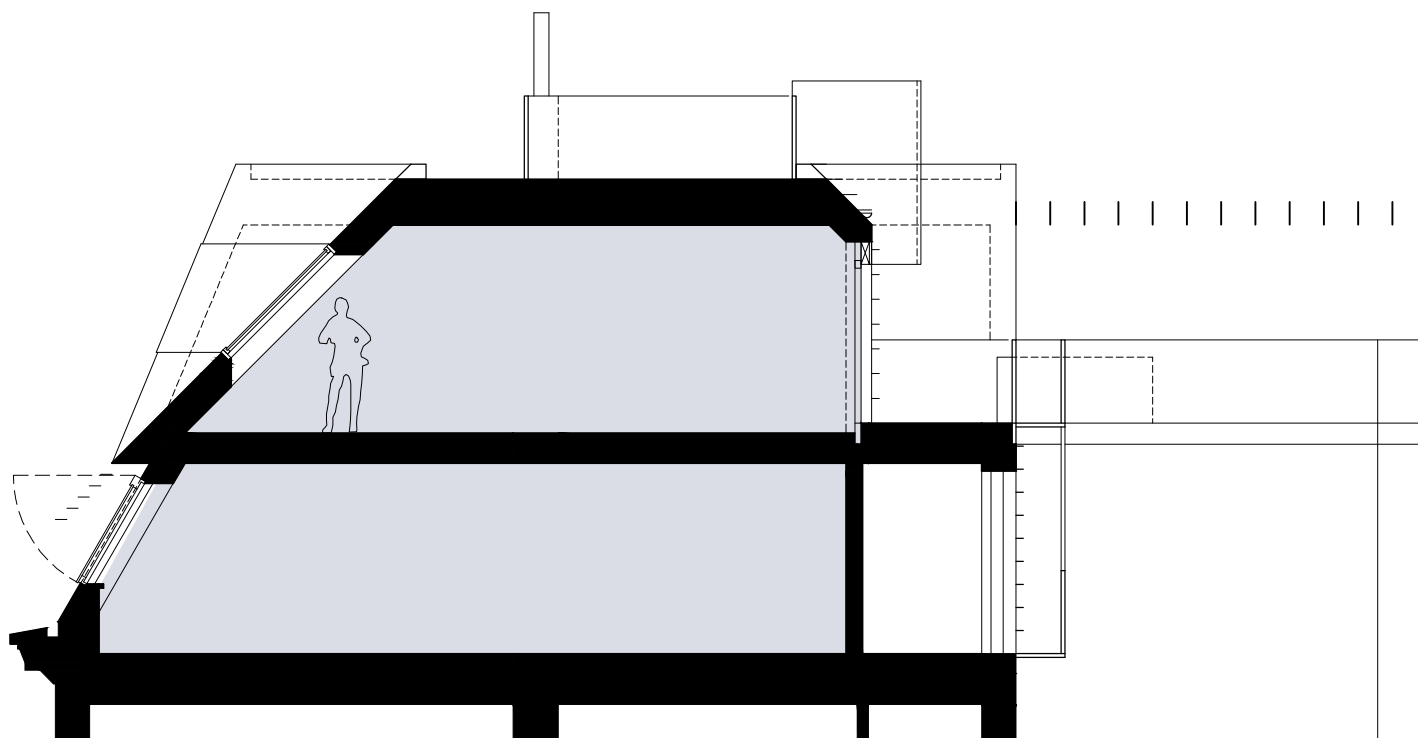
SCHNITT
