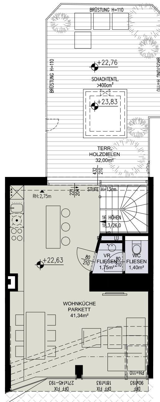
2.DG
