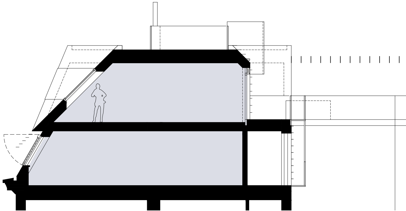
SCHNITT
