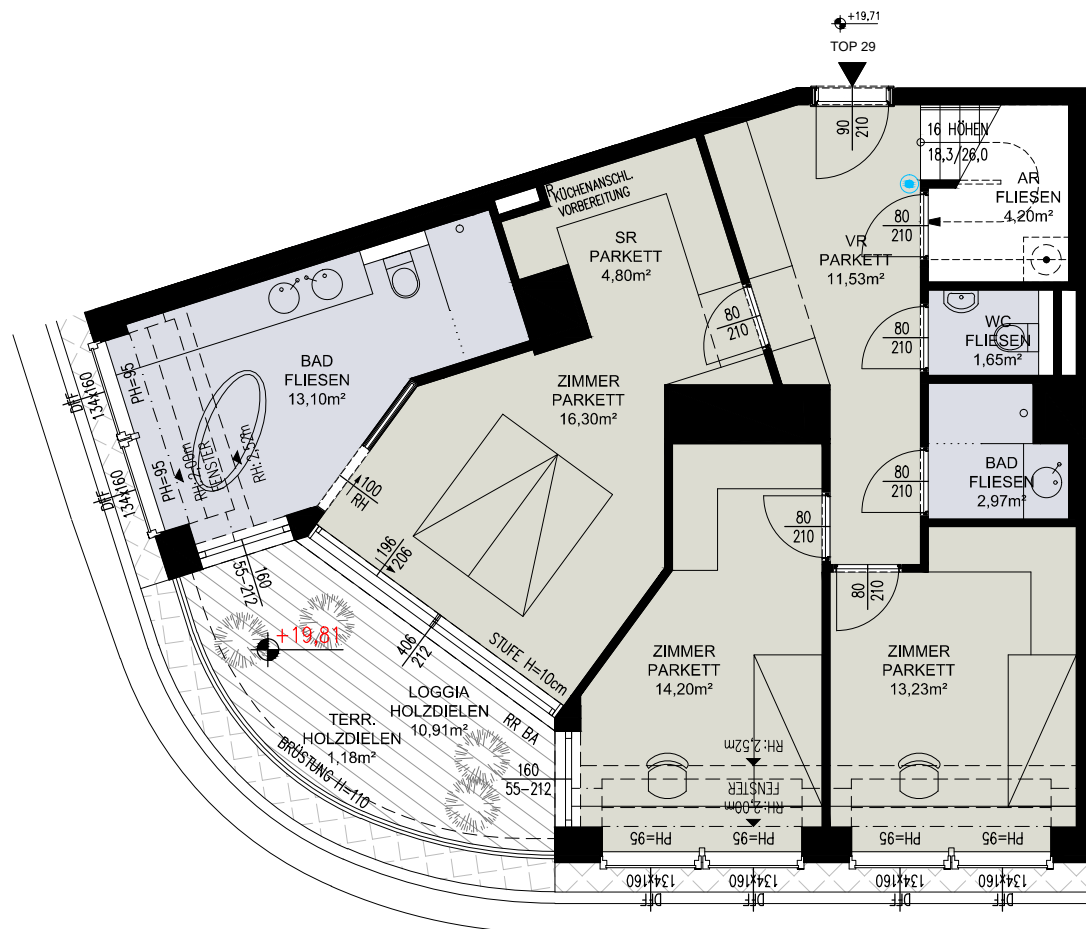
1.DG
