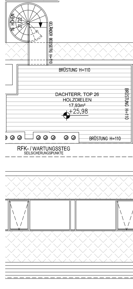
DACH
