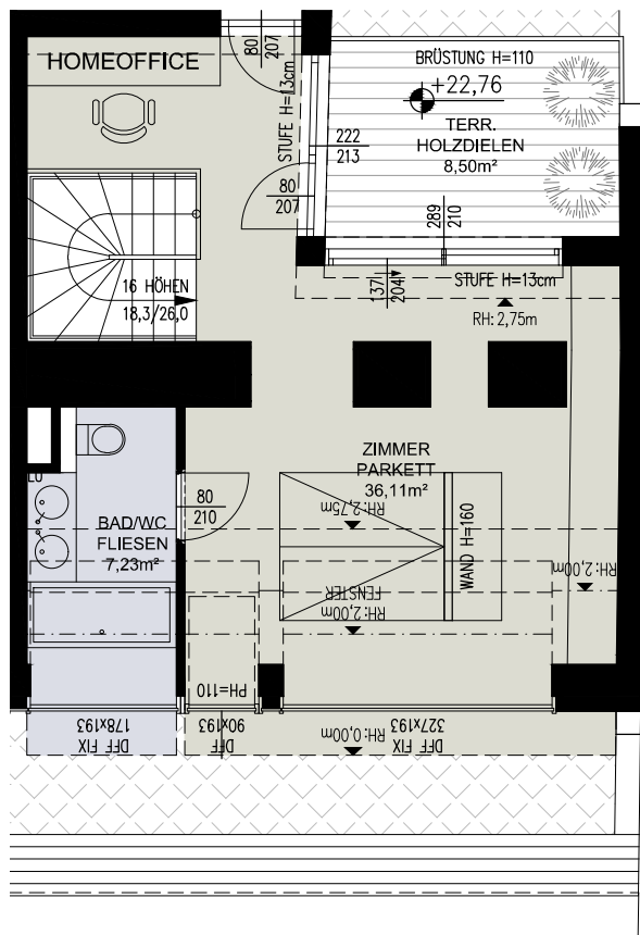
2.DG
