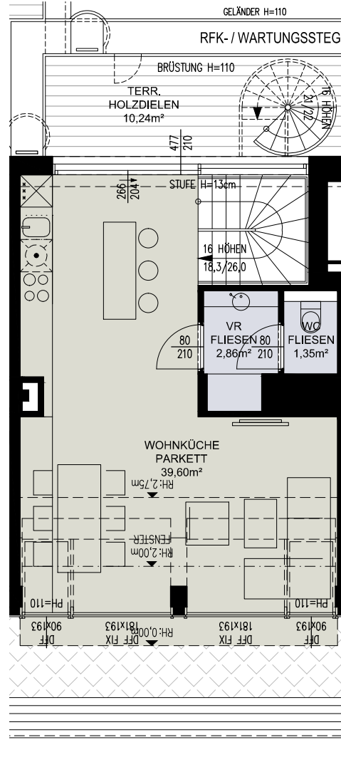
2.DG
