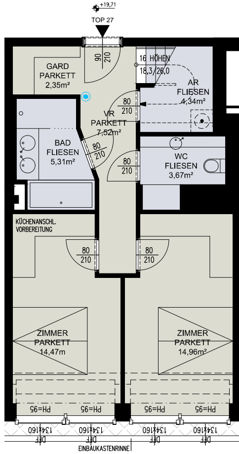
1.DG
