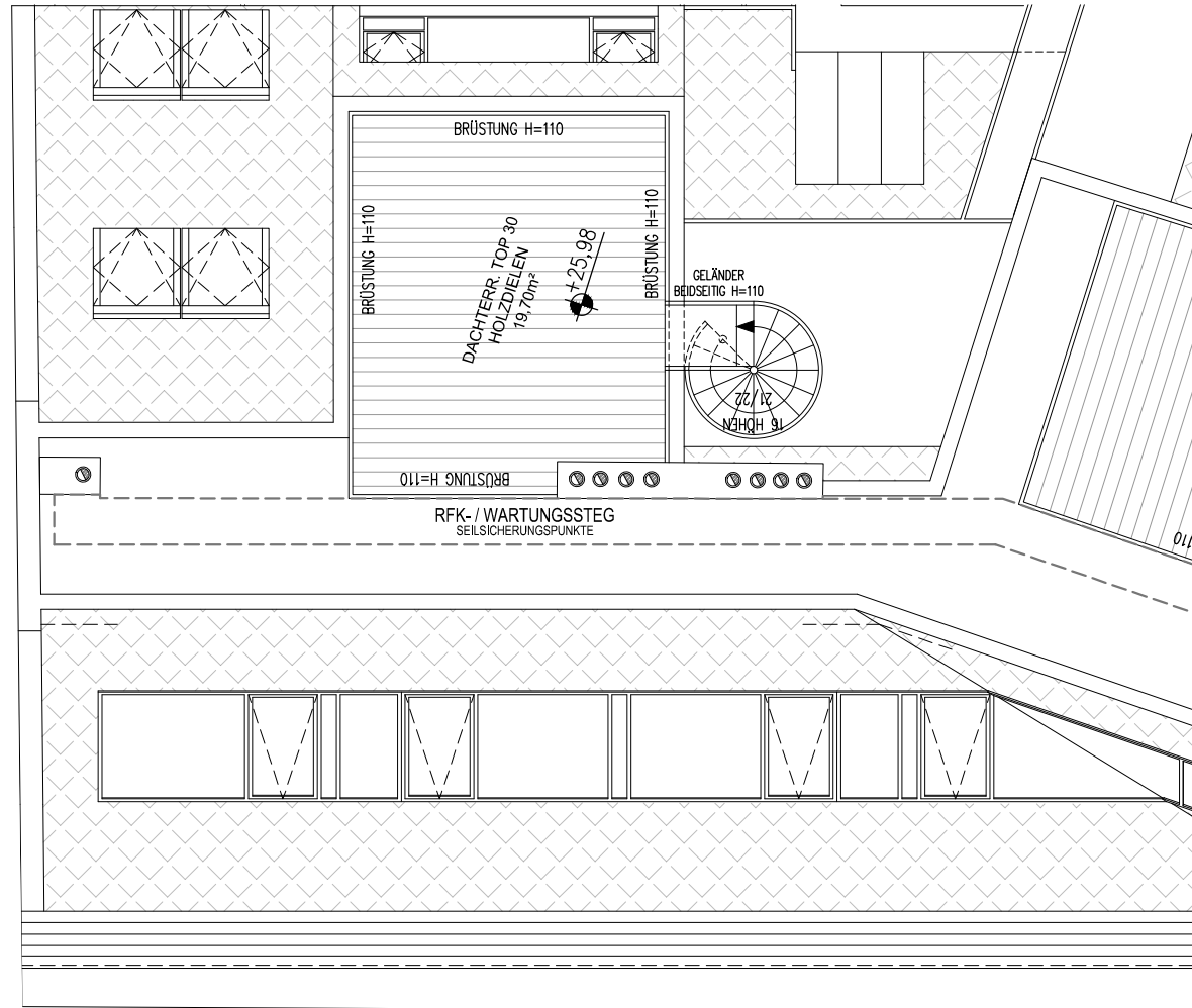
DACH
