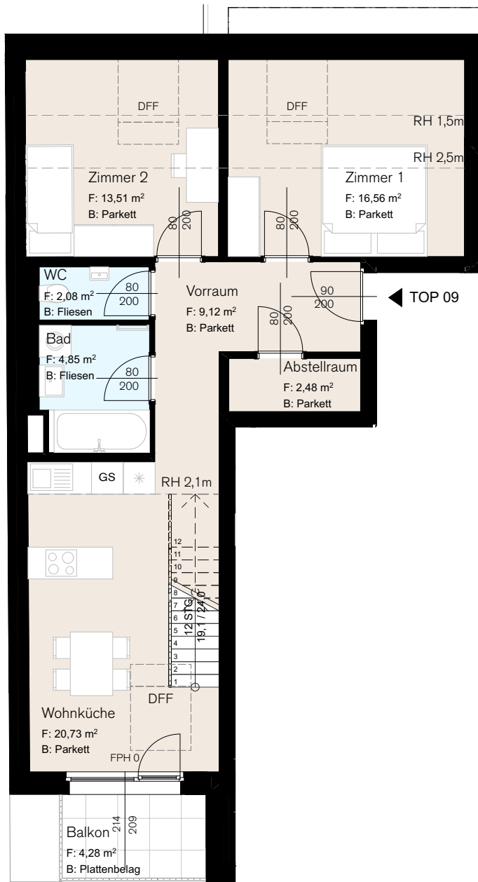
Dachgeschoss
