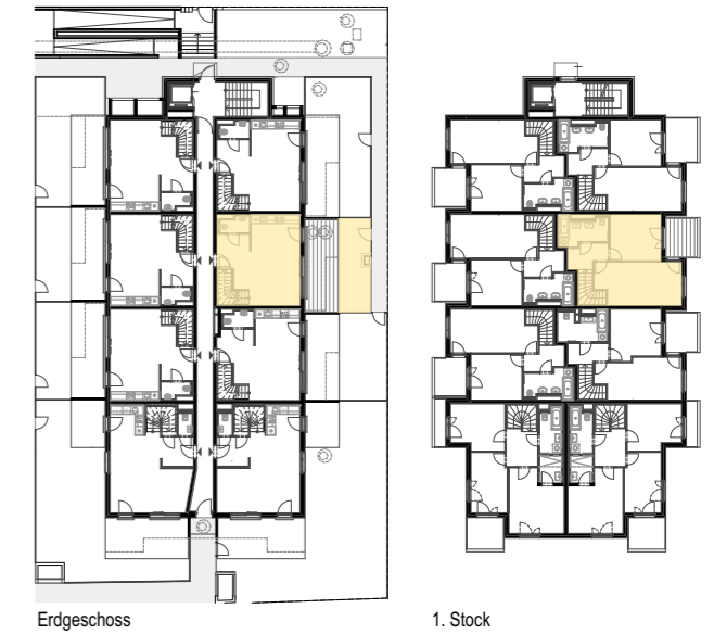
ÜBERSICHT Erdgeschoss / 1. Stock ON 11
